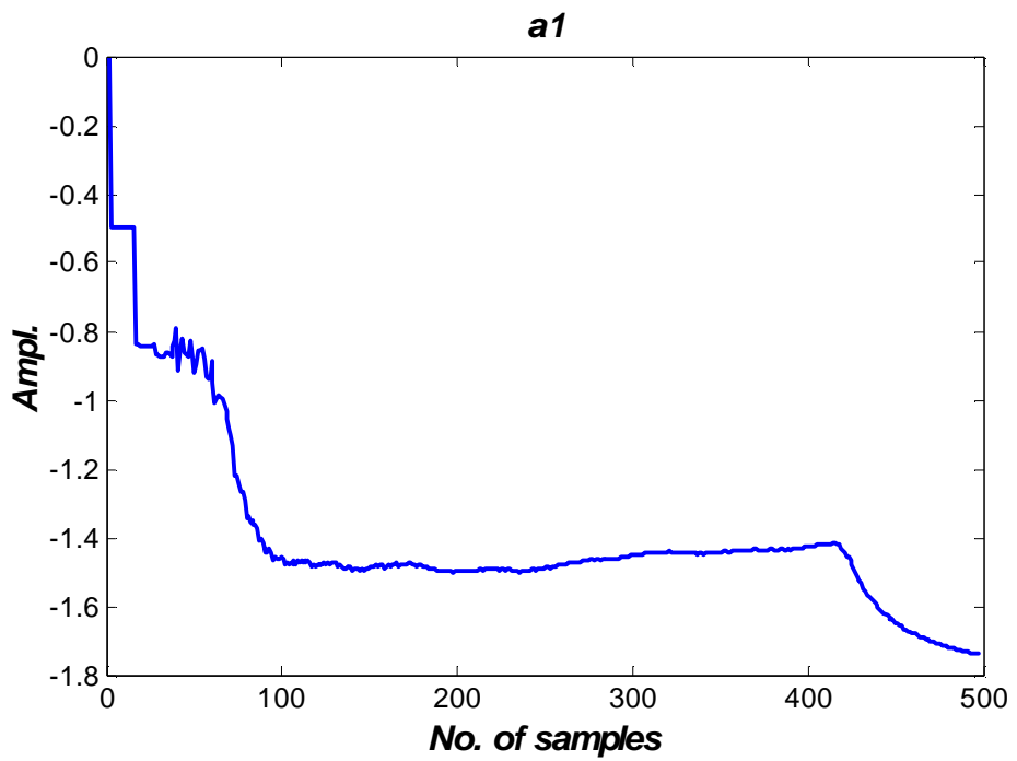
Figure (7) parameter estimate of the RLS
