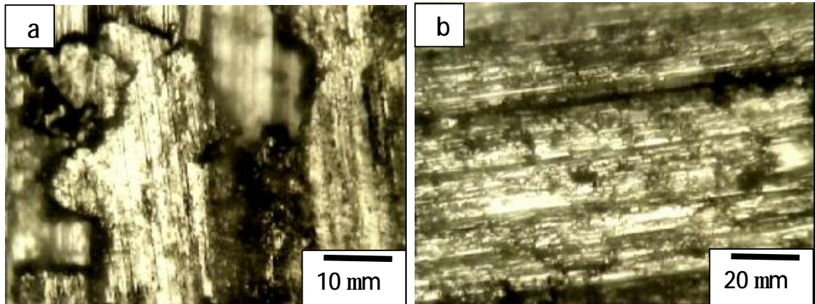
شكل (6) السطح المتأثر بالبلى عند ضغط 0.189 ميكاباسكال يوضح وجود مناطق الشقوق والإزالة للحطام من السطح على هيئة حطام معدني بسبب البلى عند أحجام أوراق كربيد سليكون مختلفة (a) 220 و (b) 120 .
