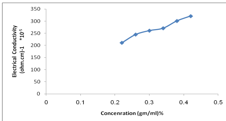
الشكل (6) تغير التوصيلية الكهربائية مع التركيز لخليط (PVA-CMC-PEG)
