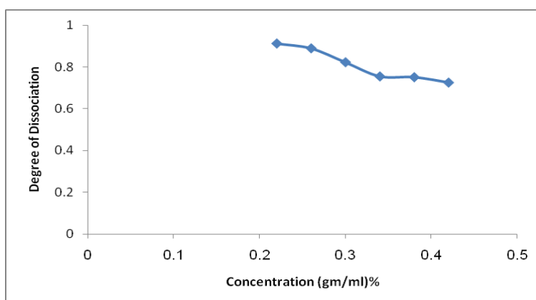
الشكل (8) تغير درجة التفكك مع التركيز لخليط (PVA-CMC-PEG)
