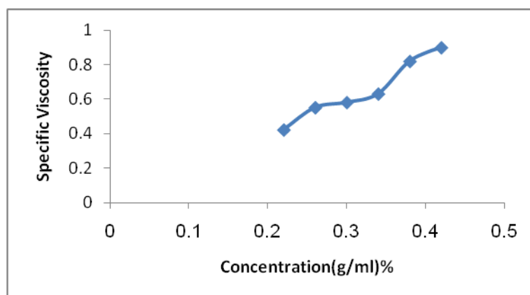
الشكل (4) تغير اللزوجة النوعية مع التركيز لخليط (PVA-CMC-PEG)
