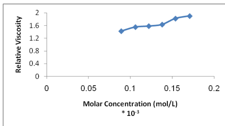
الشكل (3) تغير اللزوجة النسبية مع التركيز لخليط (PVA-CMC-PEG)
