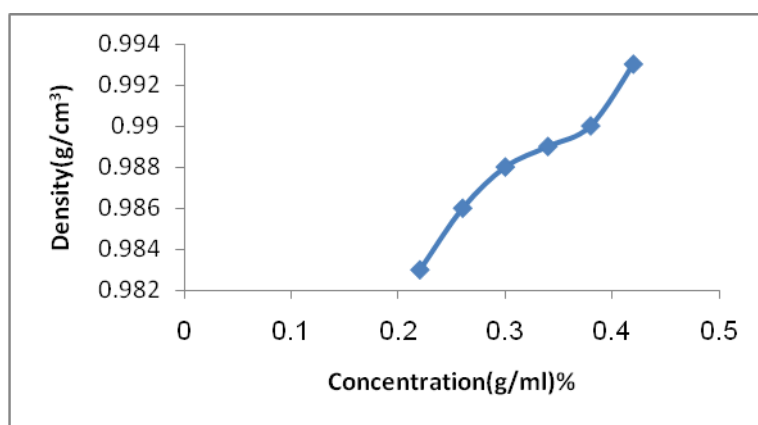
الشكل (1) تغير الكثافة مع التركيز لخليط (PVA-CMC-PEG)
