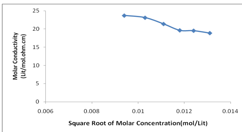
الشكل (7) تغير التوصيلية المولارية مع الجذر التربيعي للتركيز المولاري لخليط (PVA-CMC-PEG)
