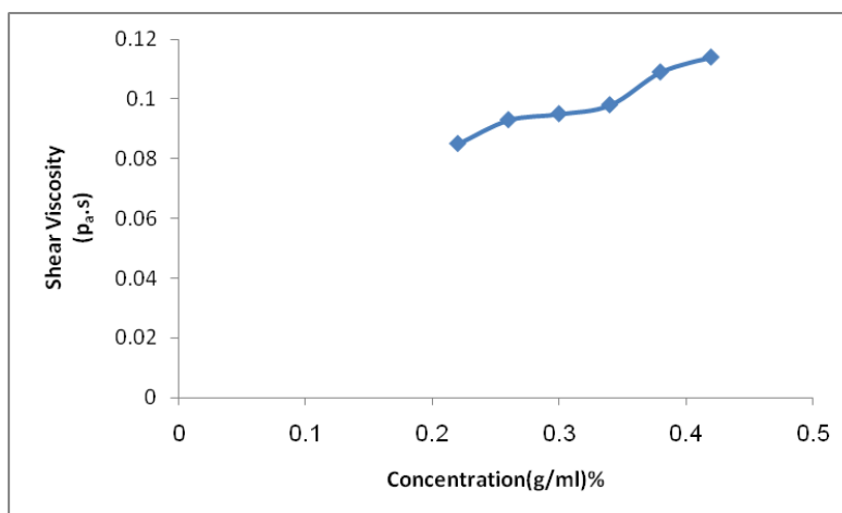
الشكل (2) تغير اللزوجة القصية مع التركيز لخليط (PVA-CMC-PEG)
