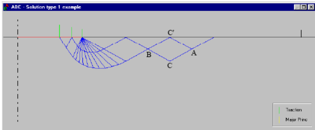
(d) CalcAB
