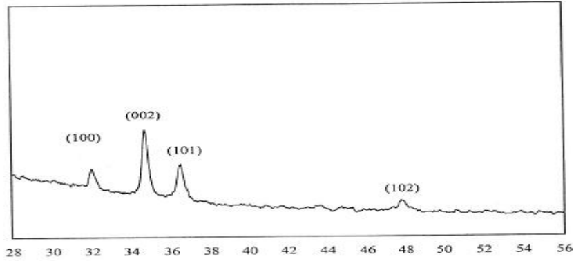
الشكل (2) طيف حيود الاشعة السينية لغشاء ZnO
