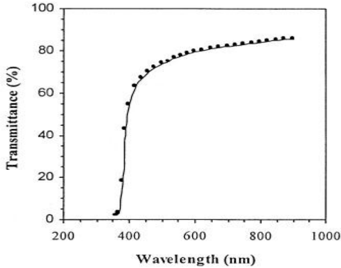
الشكل (4) تغير النفاذية كدالة للطول الموجي لغشاء ZnO
