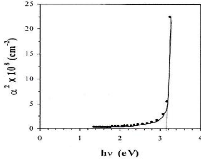
الشكل (5) حساب فجوة الطاقة البصرية الممنوعة للانتقال المباشر المسموح لغشاء ZnO
