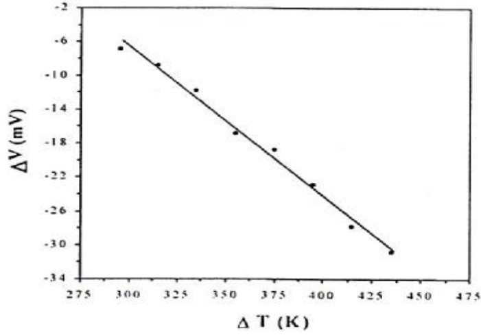
الشكل (8) تغير فرق الجهد كدالة للفرق بدرجات الحرارة لغشاء ZnO
