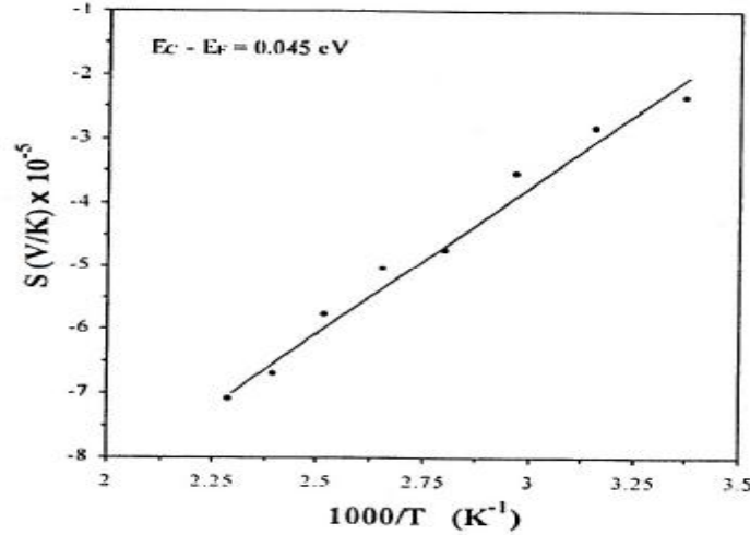
الشكل (9) تغير معامل سيبك مع مقلوب درجة الحرارة لغشاء ZnO
