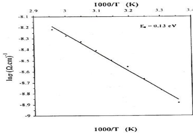
الشكل (7) العلاقة بين لوغارتم المقاومة النوعية مع مقلوب درجة الحرارة لغشاء ZnO
