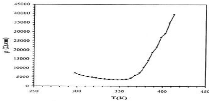
الشكل (6) تغير المقاومة النوعية كدالة لدرجة الحرارة لغشاء ZnO
